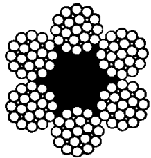
6 x 25 Filler Wire IWRC
