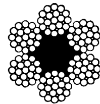
6 x 25 Filler Wire IWRC
